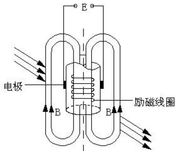
图1 工作原理
