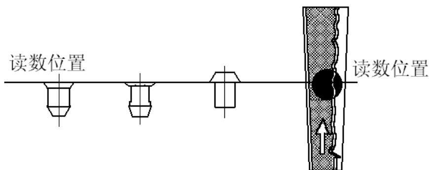
图 5 各种浮子读数位置图
