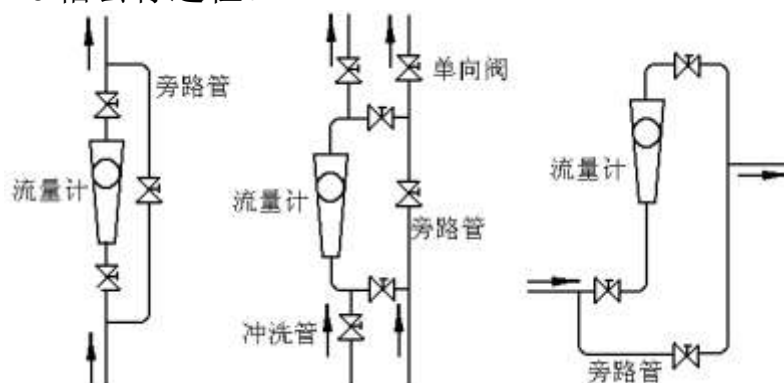
图 4 流量计安装示意图
