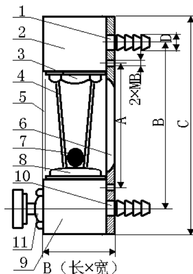
图1 DN3、DN4、DN6、DN10 结构示意图
